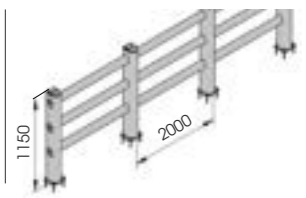
M12 VERZINKTER STAHL
